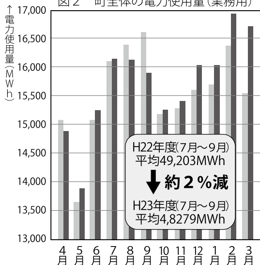
図2 町全体の電力使用量（業務用）
